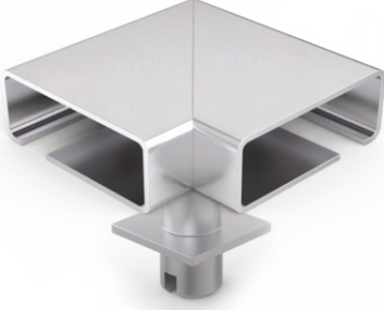
Kod : AKS 123 Ürün Adı : 60x25 Önden Kanallı Köşe Mafsal Dirsek
