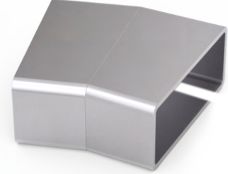
Kod : AKS 144 Ürün Adı : 80x30 135° Önden Kanallı Dirsek
