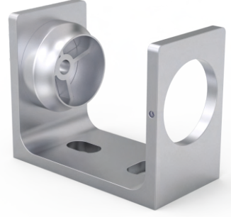
Kod : AKS 78 Ürün Adı : 35' lik Dikme Yandan U Bağlantı
