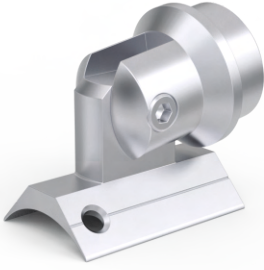
Kod : AKS 01 Ürün Adı : 35°' lik Mafsal Takımı 4 Alyan
